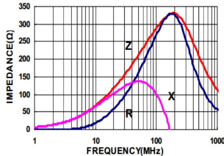
CVB2012P301T
